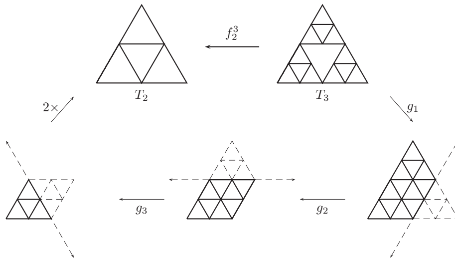
Figura 2. La función f_2^3 paso a paso.
