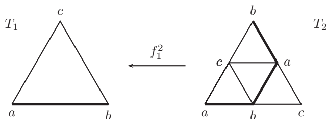
Figura 3. (f_1^2)^{-1}(ab) , (f_1^2)^{-1}(bc) y (f_1^2)^{-1}(ac) son arcos.
