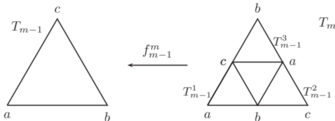
Figura 4. Codificacion de los grafos T_{m-1} y T_m .
