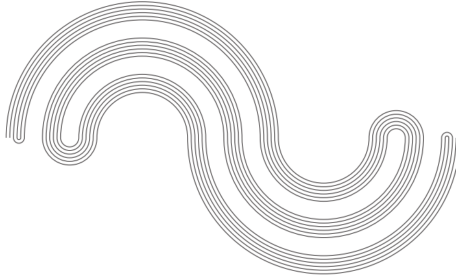
Figura 5. Continuo de Knaster con dos puntos finales.
